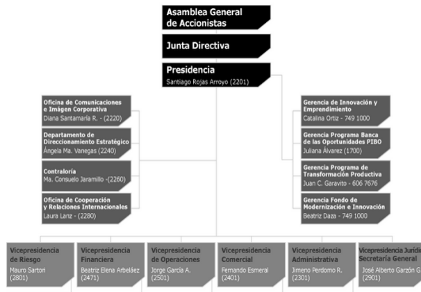
Gráfico 8: Estructura Organizacional
